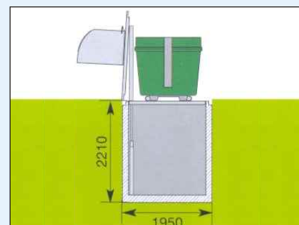
Medidas de la Ref. CS.L01 (vista lateral)
