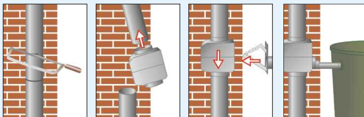
Instalación simple y rápida en tres pasos, cortando el tubo de la canal y acoplando el filtro
