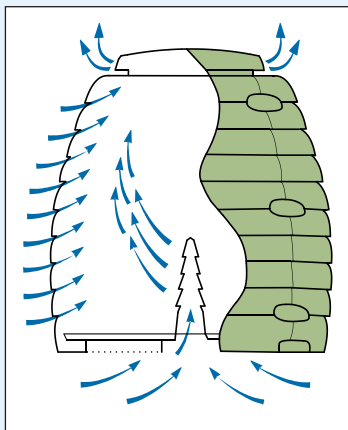
Ventilación del compostador
