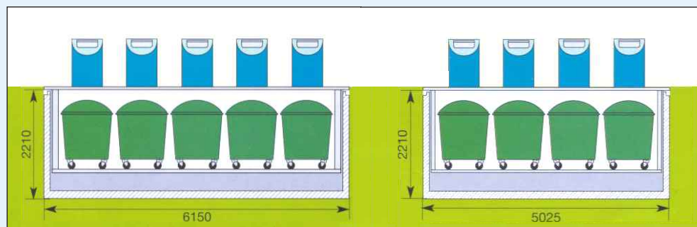
Medidas de la Ref. CS.H05
