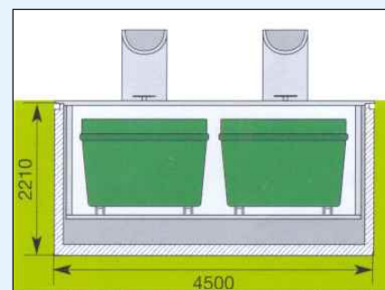
Medidas de la Ref. CS.L02 (vista frontal)
