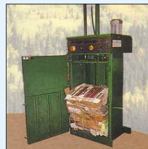
Bala de cartón resultante
