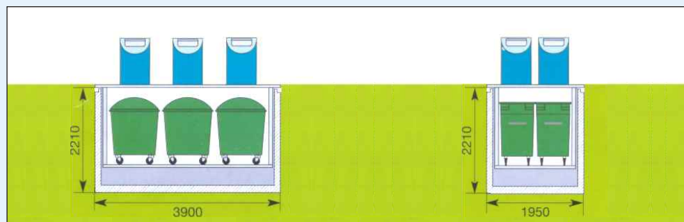
Medidas de la Ref. CS.H03
