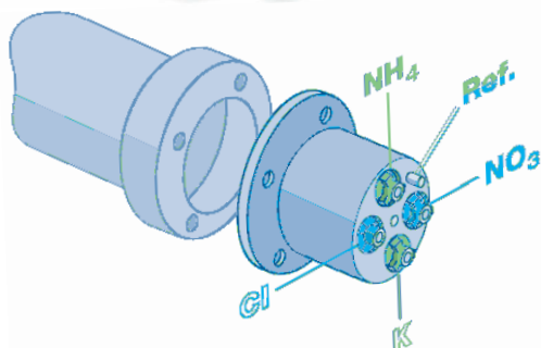
Cartucho CARTRICAL plus para amonio ( \text{NH}_4 ) y nitrato ( \text{NO}_3 ), con compensación de cloruro (Cl) y potasio (K)
