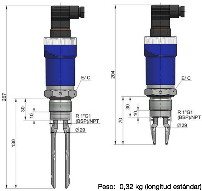
LD60 / LD61 - Conexión roscada BSP / NPT
