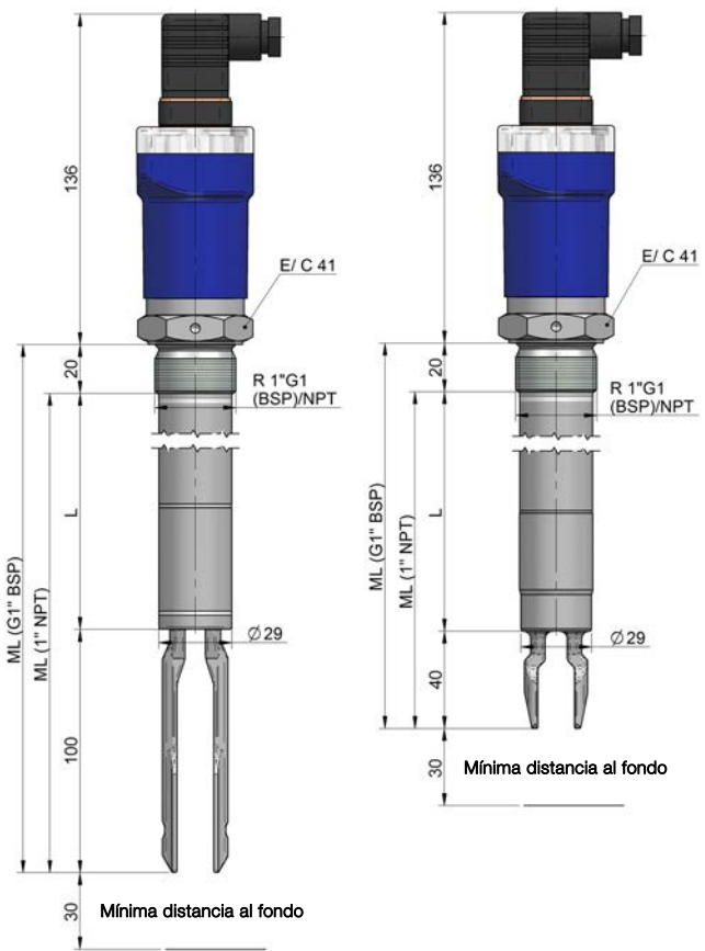
LD60ML / LD61ML - longitud especial
