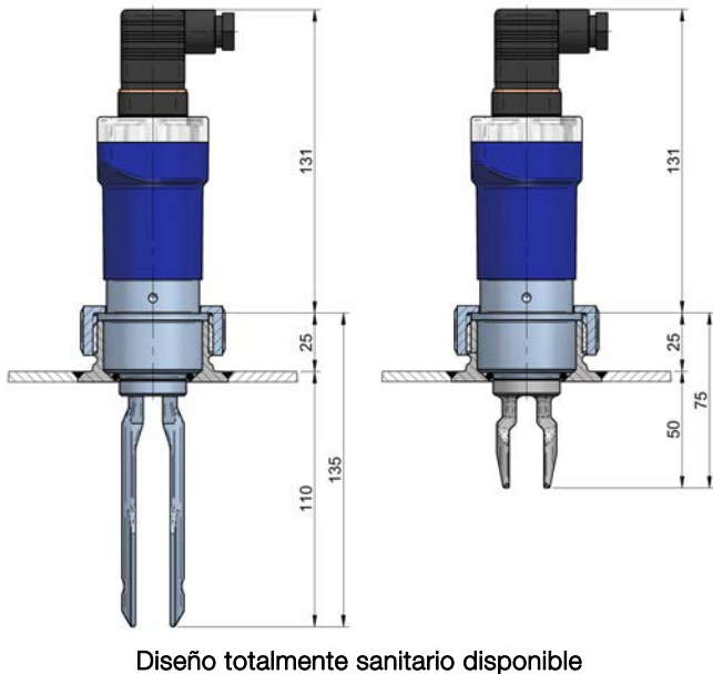
LD60 / LD61 - Conexión nivelada TF DIN405
