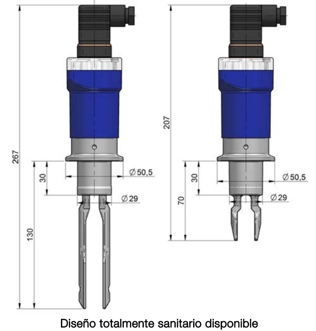
LD60 / LD61 - Conexión CLAMP ISO 2852
