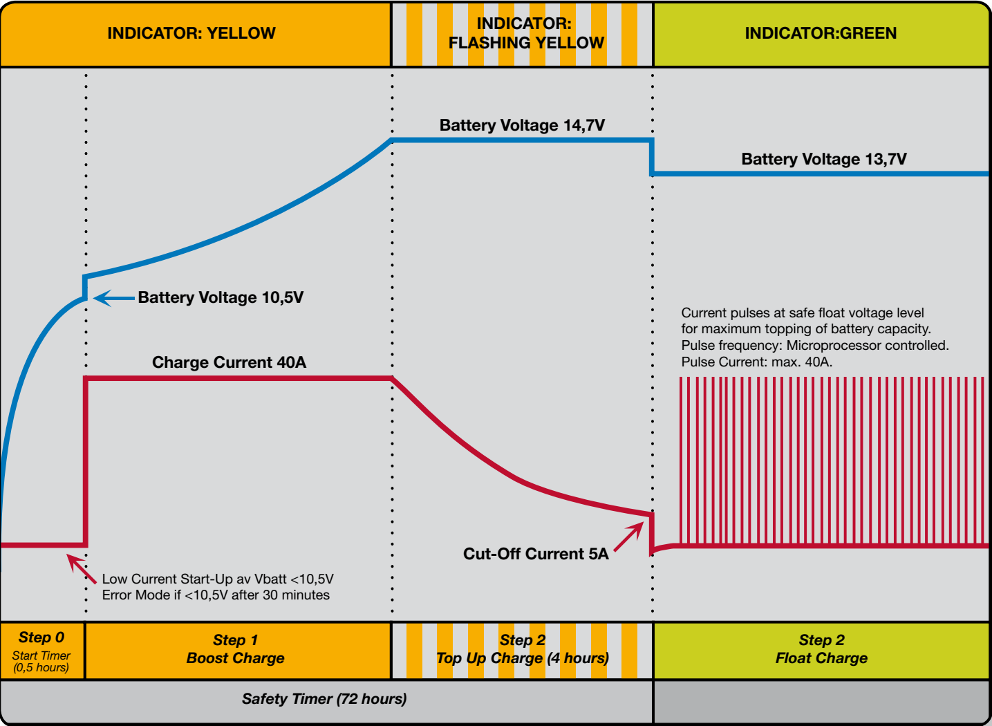
Charging characteristics and LED indication / Ladekarakteristikk og lysdiode (LED) indikasjon (data for model 2245 - 12V version)
