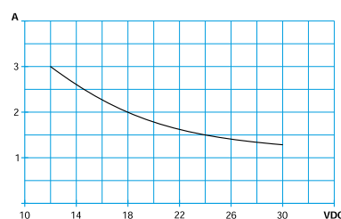
12-30 VDC version / 12-30 VDC versjon
