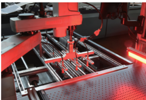
Equipado con el robot de visión binocular YAMAHA con una precisión de 0,1 mm.
