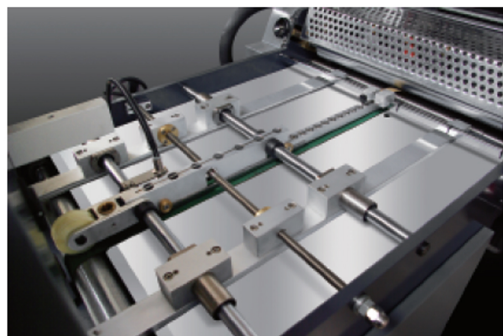
El Alimentador automático no causa deformación en el papel.
