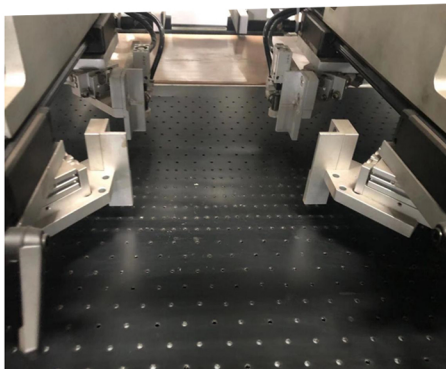
Pieza formadora de caja automática. Dispositivo de sujeción de caja automático anti-fricción (elevación de 15 mm)
