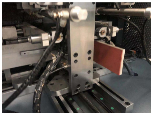
Estructura general de elemento de presión
