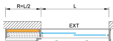
2 hojas (sobre 2 raíles) Apertura a la izquierda
