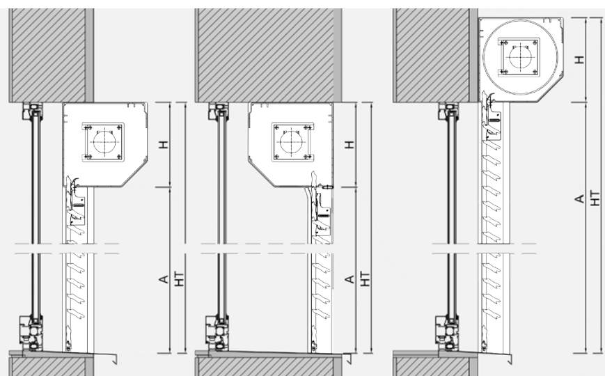
En.exterior: intra-muro
