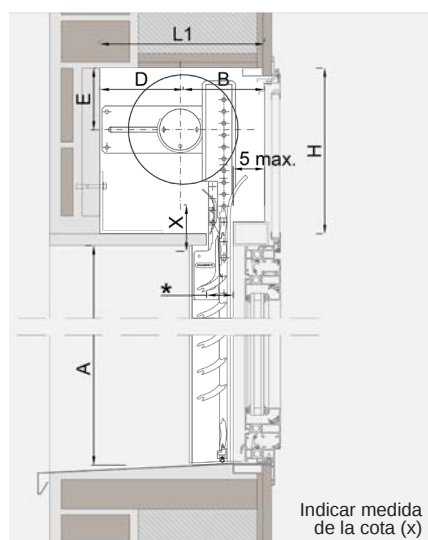
Enrollamiento exterior
