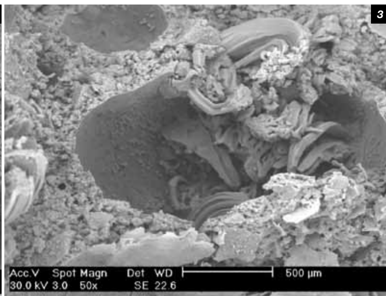
foto 2 – Macroporos presentes en los morteros deshumidificantes de la línea MAPE-ANTIQUE
