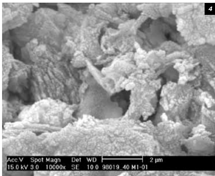
foto 5 – Microfotografía con microscopio electrónico, de un mortero MAPE-ANTIQUE transcurridos 8 días de “envejecimiento”. Se nota la estructura redondeada típica de un sistema estabilizado
