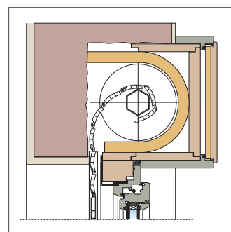
revestimiento y aislamiento del cajón de persiana
