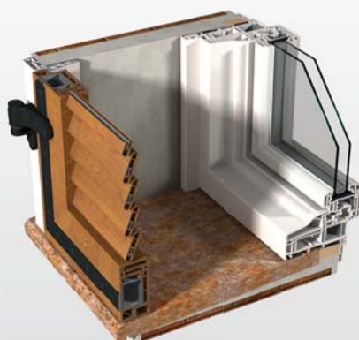
Ventana de renovación mallorquina con marco de solape exterior
