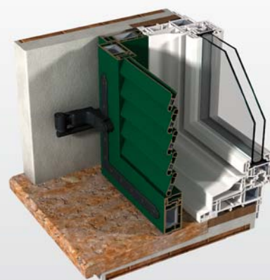
Obra nueva marco Bloc mallorquina con marco y herrajes con saliente
