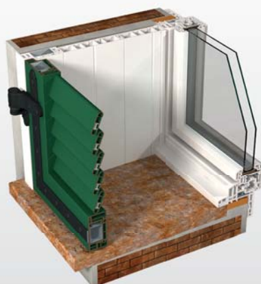
Ventana de renovación mallorquina con marco de revestimiento pared
