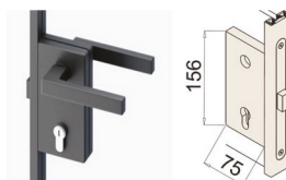
⑪ CERRADURA VERTICAL MAGNÉTICA CON LLAVE
