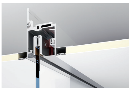
FALSO TECHO SIN DINTEL
