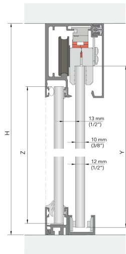
INSTALACIÓN VISTA ROLLGLASS 150 TOP
