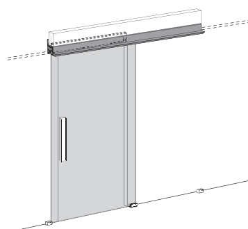
UNIKGLASS + EMPOTRADO SIN DINTEL
