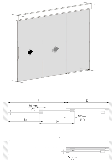
Extendo 2 hojas con vidrio fijo
