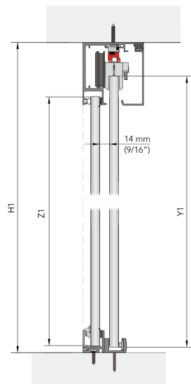
INSTALACIÓN VISTA ROLLGLASS 250
