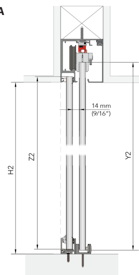
INSTALACIÓN EMPOTRADA ROLLGLASS 250
