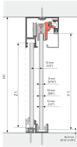
INSTALACIÓN VISTA ROLLGLASS 50/100
