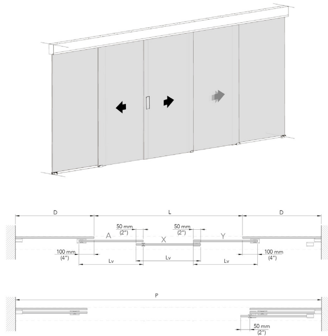
Extendo 3 hojas con vidrio fijo
