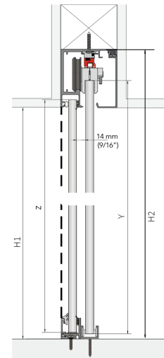
INSTALACIÓN EMPOTRADA ROLLGLASS 150 TOP
