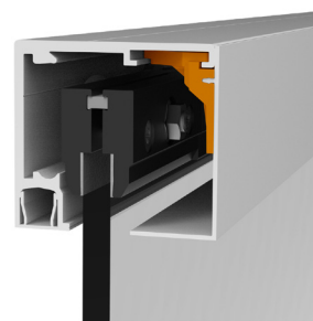
Clip para tapeta con geometría pensada para reforzar la rigidez de la tapeta.
