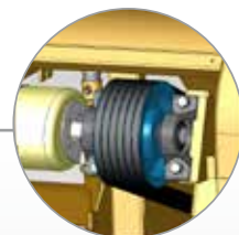
transmisión con correa múltiple con tensor de resorte y embreague de seguridad
