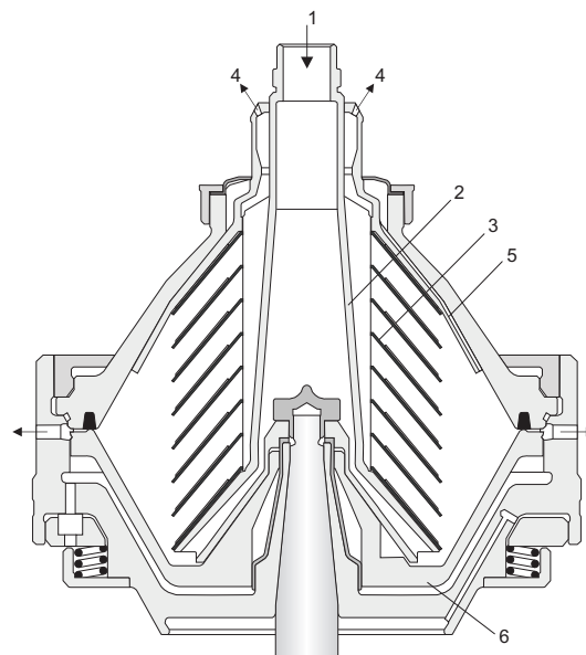
Fig. 2 Plano de una cuba típica de una centrifugadora de extracción de sólidos. Es posible que los detalles del plano no se correspondan con la centrifugadora descrita.
