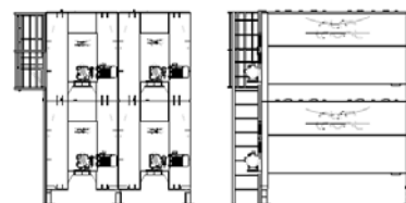
ALFABAT 4004 - BATIDORA CUADRUPLA
