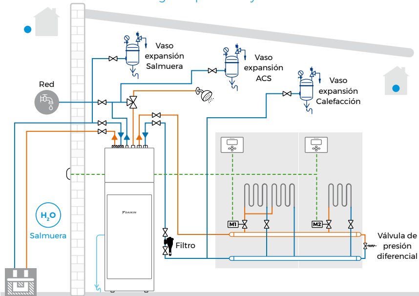
Ejemplo Daikin Altherma GEO con depósito integrado para ACS y suelo radiante*
