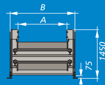
SECCIÓN A-A
