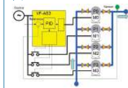
Ejemplo de sistema de controlador de varias bombas
