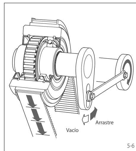
La fig. 5-6 muestra una rueda libre de avance, en la que el aro exterior realiza el movimiento de vaivén y el exterior el movimiento de avance paso a paso.
