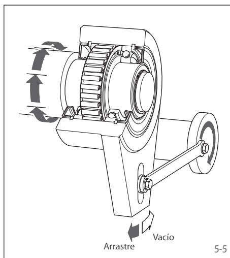
La fig. 5-5 muestra una rueda libre de avance, en la que el aro interior realiza el movimiento de vaivén y el interior el movimiento de avance paso a paso.
