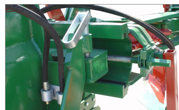
Detalle cabezal desplazable
