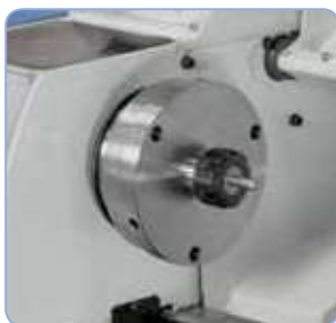
El portapinzas ER 25 asegura una alta concentricidad de amarre, pinzas desde 1 a 16mm.
