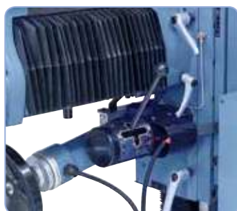
Palanca de selección de eje de movimiento (en la imagen para X y Z), ajuste de la velocidad de avance mediante potenciómetro en el panel de control
