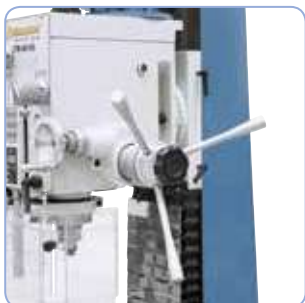
Ajuste fácil de la pinola a la hora de taladrar gracias a manijas dispuestas de forma ergonómica. Volante con escala para un ajuste preciso a la hora de fresar
