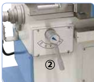
1: Palanca de selección de la dirección de avance 2: Palanca de selección de avance de eje
