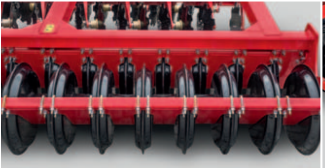
Compactador doble SteelDisc para una consolidación óptima también en suelos muy pesados
