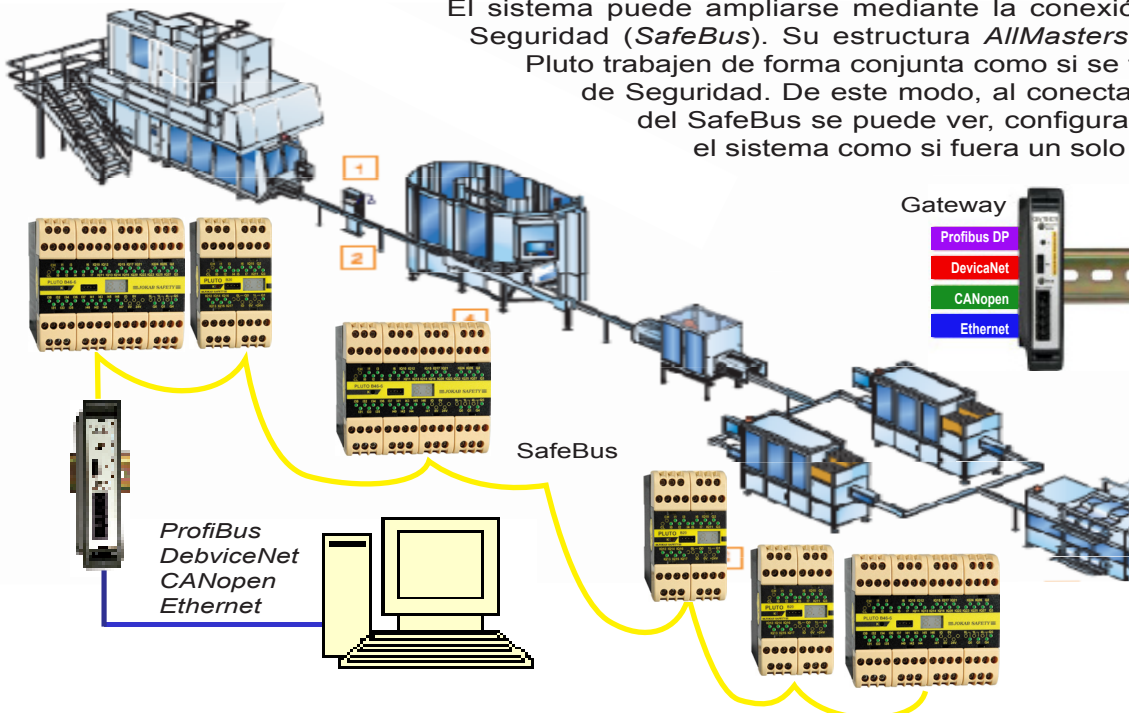
Pluto B46-6 34 E/S + 6S Seguridad
