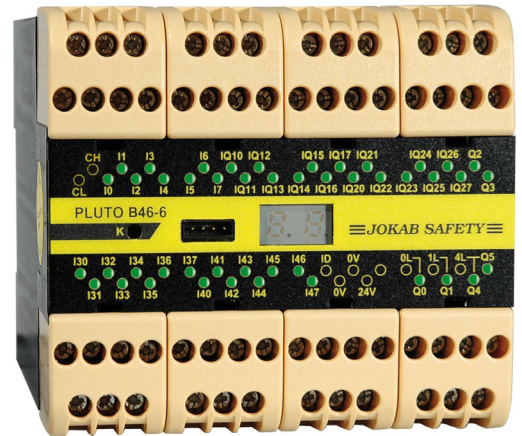
Pluto B46-6 34 E/S + 6S Seguridad
