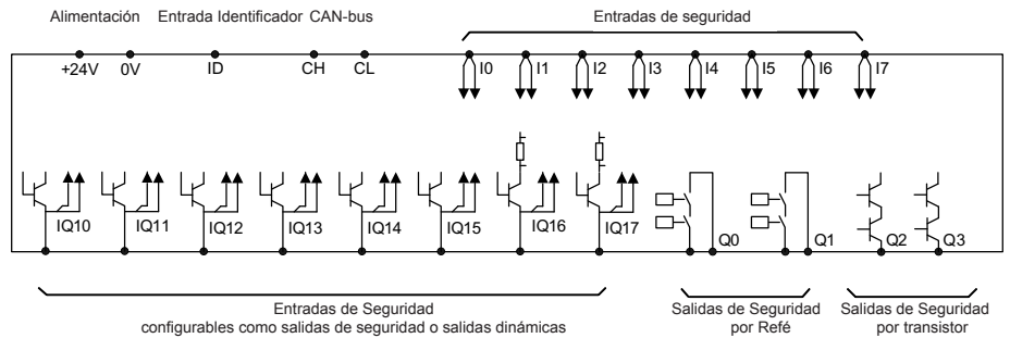
Pluto B20 16 E/S + 4S Seguridad
