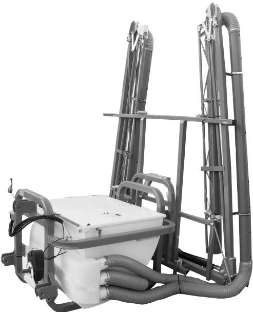
Mod. Barra hidráulica
