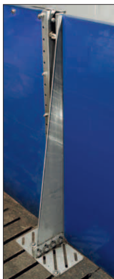
Poste refuerzo
