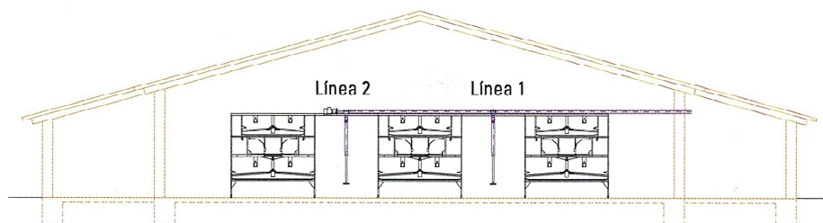
Sección transversal de la nave: PickPuck con llenado automático
