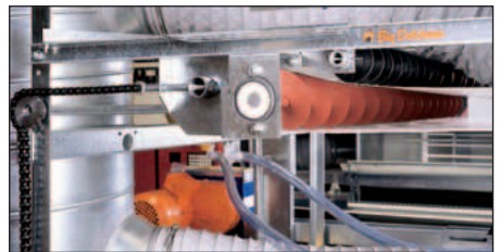
Unidad terminal de basura con rodillo limpiador
