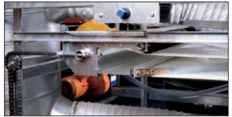
Unidad terminal de basura (estándar)
