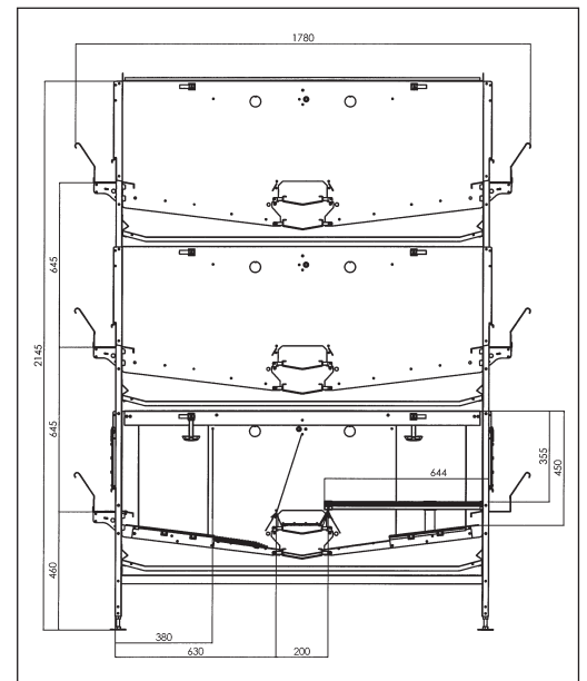
Sección de una AVIPLUS de 3 pisos
