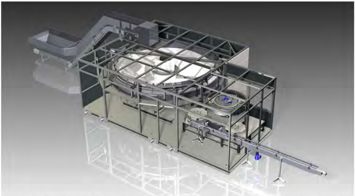
Interior de MONOCHUTE-50 con Orientador Rotativo incorporado en monoblock. (Simulación 3D).
