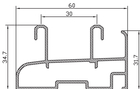
MARCO 60 CON REGISTRO 15201
