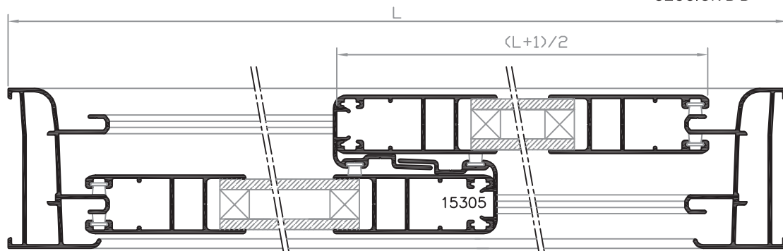
SECCIÓN B-B'
