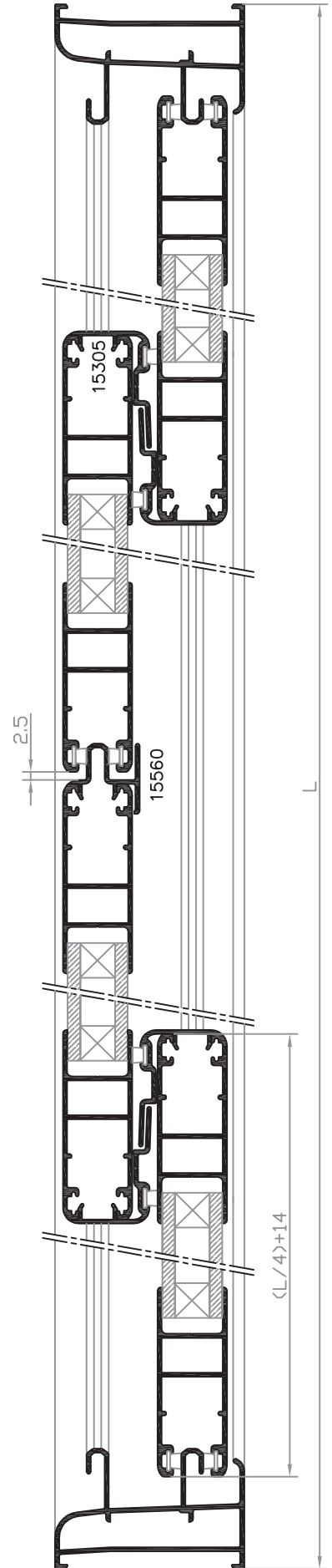
SECCIÓN B-B'
