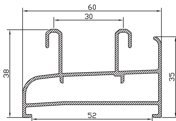
MARCO 60 CON CLIP 15200
