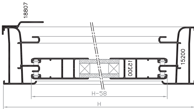
SECCIÓN A-A'
