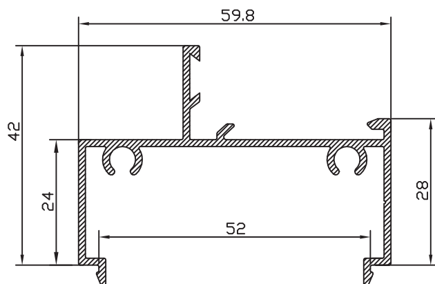
MARCO FIJO MACHO 2000 02263
