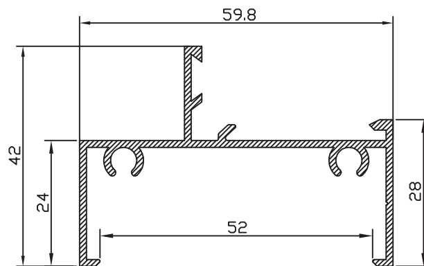
MARCO FIJO HEMBRA 2000 02264
