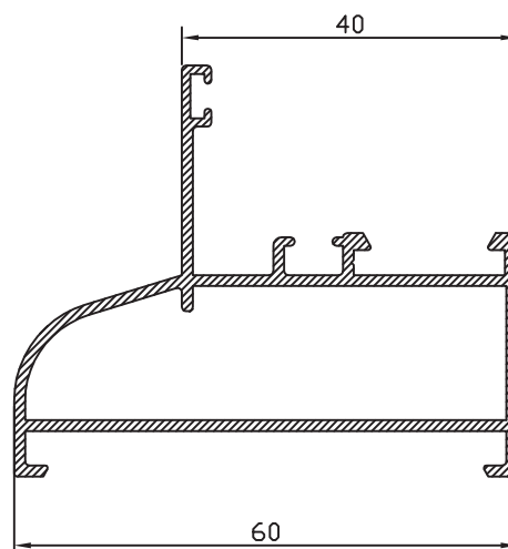
MARCO FIO CON CLIP 28272
