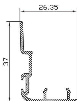
CLIP DE CIERRE 15305
