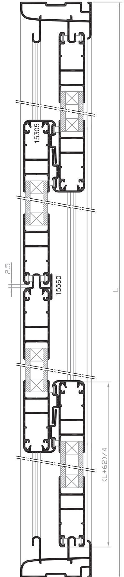
SECCIÓN B-B'
