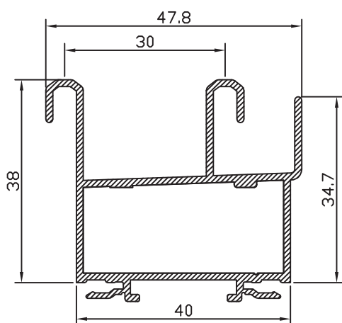
MARCO 40 CON CLIP LATERAL *15203
