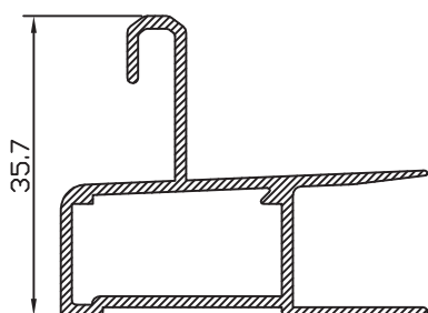
ACOPLE TRES CARRILES 15202
