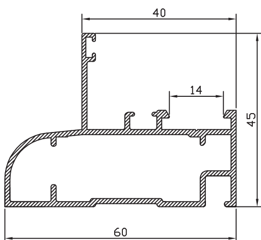
MARCO FIJO CON REGISTRO 28271
