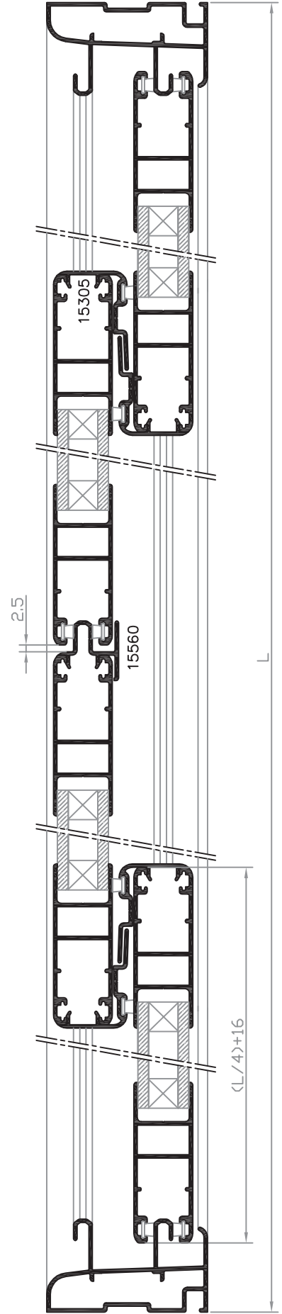
SECCIÓN B-B'
