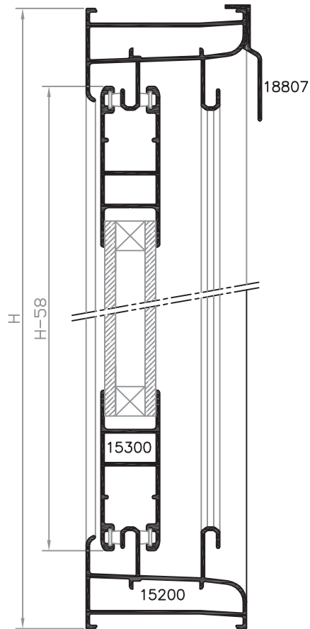
SECCIÓN A-A'
