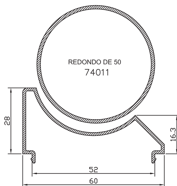
REDONDO DE 50 74011 ESQUINERO REGULABLE 21725
