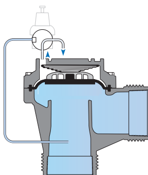
Posición abierta
