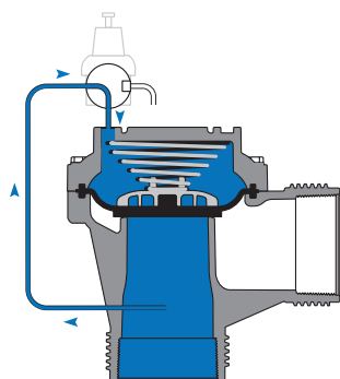
Posición cerrada
