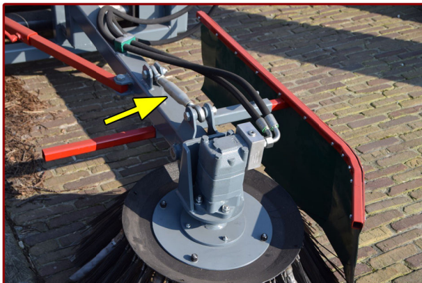
▲ Inclinación vertical del cepillo ajustable manualmente Manually Adjustable Brush Vertical Tilt
