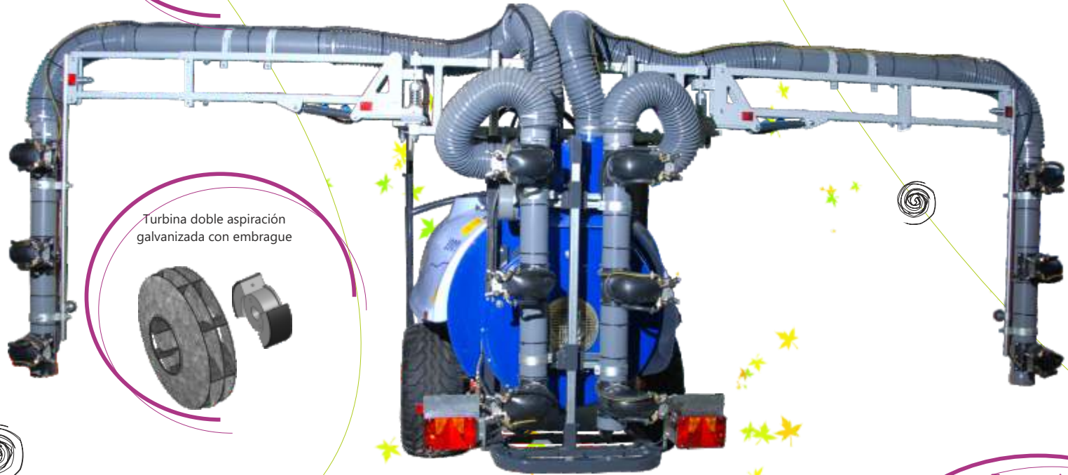
Movimiento brazos hidráulicos: subir/bajar; abrir/cerrar individual; levantar brazo para salvar hilera
