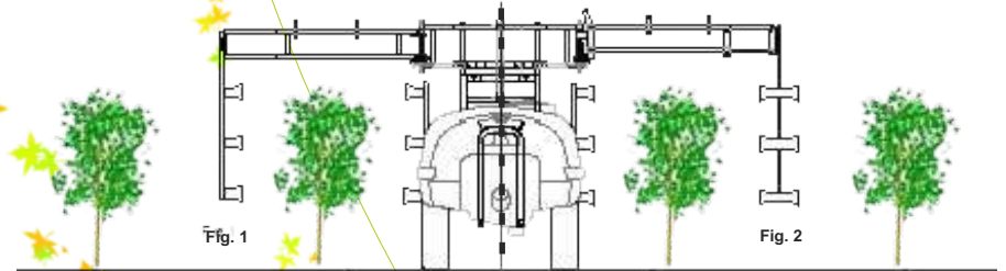
Movimiento brazos hidráulicos: subir/bajar; abrir/cerrar individual; levantar brazo para salvar hilera
