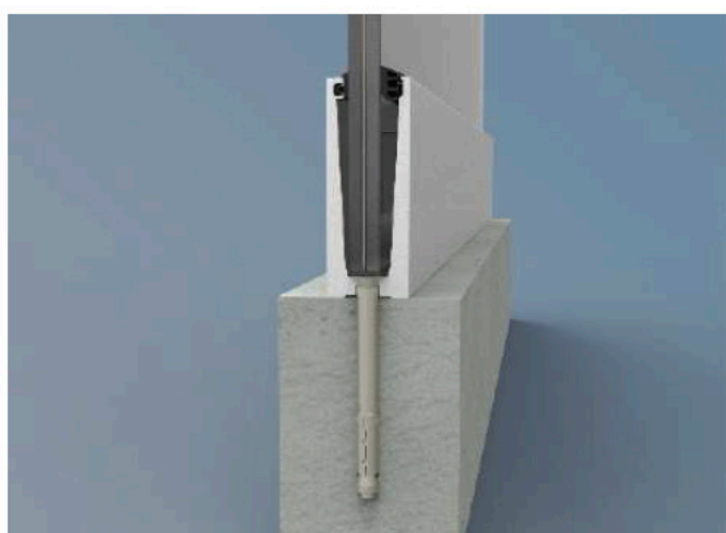
Fijación. Su sistema de anclaje de alta tecnología le garantiza la máxima eficiencia y seguridad .
