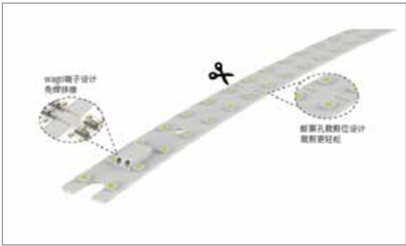
硬板模组 铝基板专配模组光源，出光均匀，散热更佳。 Wago 免焊端子，可便捷拼接。
