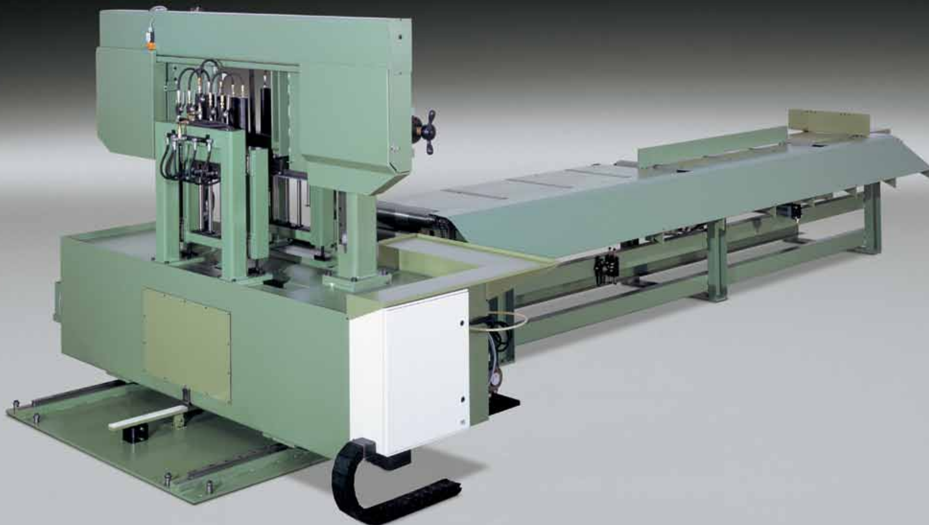
Línea de corte en colada continua de bronce y latón. Descarga hasta 4 m.
