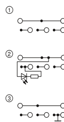
13,5 A, borne de cuatro conductores para actuadores
