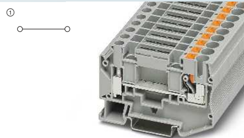
52 A, borne de paso, de igual contorno
