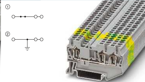
17,5 A, borne de paso, 3 conexiones
