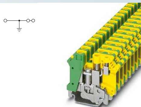
10 (16) mm 2 , 76 A, borne de tierra con auto-gobierno y pie PE
