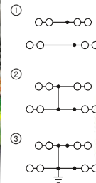
24 A, borne de doble piso, 4 conexiones por piso
