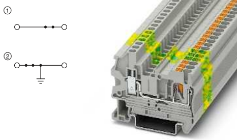
24 A, borne de paso
