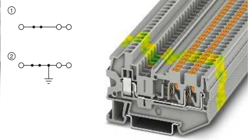
24 A, borne de paso, 3 conexiones
