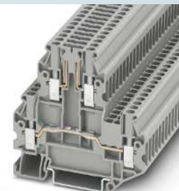
24 A, borne de doble piso con zona de interrupción
