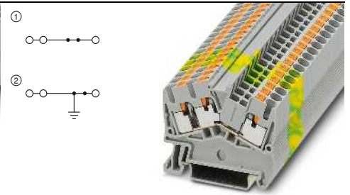
28 A, borne de paso, 3 conexiones
