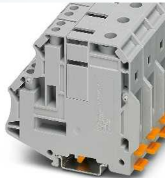
192 A, borne colectivo de potencial, 4 entradas de 10 mm 2
