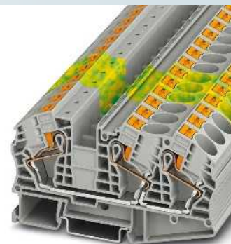
85 A, borne de paso, 3 conexiones
