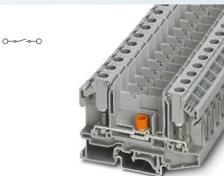
6 (6) mm 2 , 41 A, borne seccionable, con hembras roscadas para tomas de prueba, para alojar puentes de conmutación
