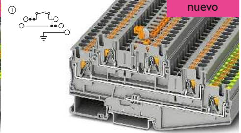
20 A, borne de tres pisos con cuchilla seccionadora
