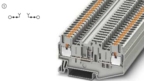
16 A, borne seccionable, con 4 fosos funcionales
