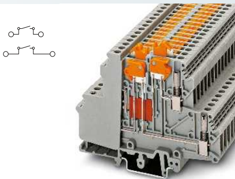
4 (4) mm 2 , 10 A, borne de doble piso, cuchilla seccionadora por piso, hembra roscada para tomas de prueba
