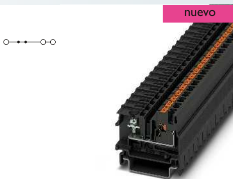
24 A, borne de paso, conexión push-in en un lado
