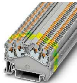
17,5 A, borne de paso, 4 conexiones
