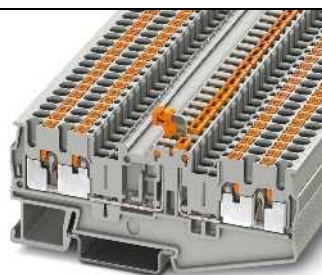
16 A, borne interrumpible por cuchilla, 4 conexiones, 4 fosos funcionales
