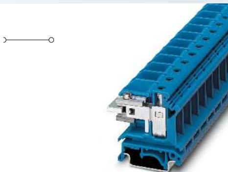
16 (25) mm², 90 A, borne de separación N
