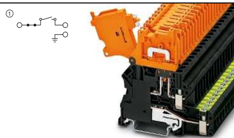
20 A, borne interruptible por palanca, de igual contorno, con pie PE
