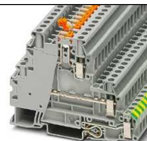
36 A, borne de varios pisos con zona de interrupción por cuchilla, pie PE
