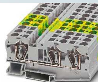
52 A, borne de paso, 3 conexiones
