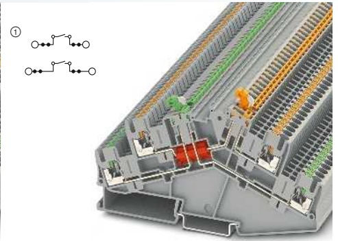
16 A, borne de doble piso con cuchilla seccionadora por cada piso, ejecución para sobremesa
