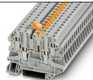
20 A, borne interrumpible por cuchilla, 4 conexiones
