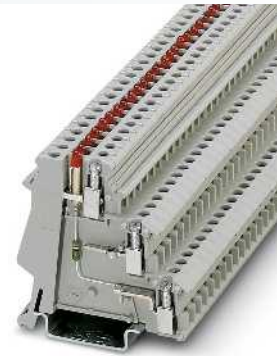
2,5 (4) mm 2 , 26 A, borne de tres conductores con indicador luminoso
