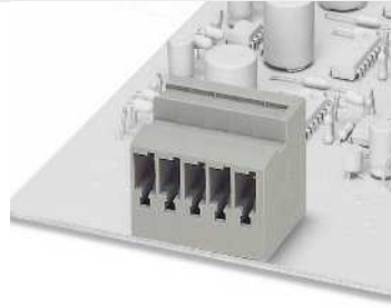
32 A, carcasa de base, sentido de conexión horizontal
