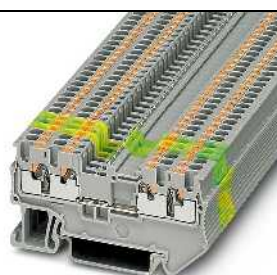
17,5 A, borne de paso, 4 conexiones
