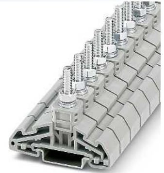
35 (35) mm 2 , 125 A, M6 borne de espárrago
