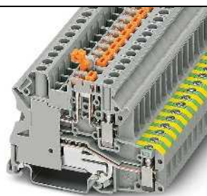
20 A, borne interrumpible por cuchilla con pie PE
