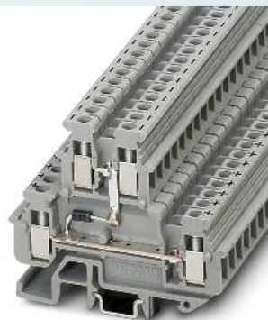
2,5 (4) mm 2 , 24 A, borne de doble piso, con diodo incorporado 1N 4007
