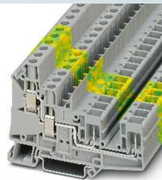
41 A, borne de paso, 4 conexiones
