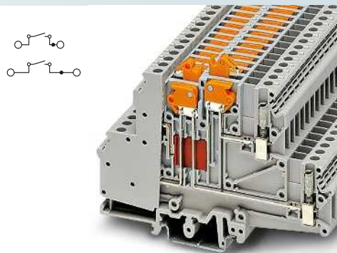
4 (4) mm 2 , 10 A, borne de doble piso, cuchilla seccionadora y entrante de puente por piso, hembra roscada para tomas de prueba
