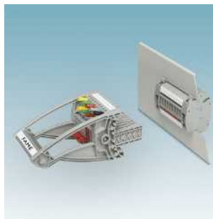
FAME 1: sistema enchufable de prueba con conector de servicio y cortocircuito del transformador en la regleta de clavijas de prueba
