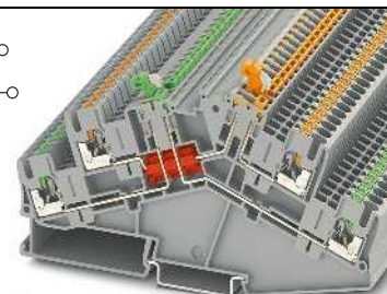
16 A, borne de doble piso con cuchilla seccionadora para sobremesa
