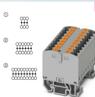
24 A, montaje sobre carril NS 15, longitudinalmente respecto al carril
