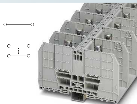
300 (300) mm 2 , 520 A, borne de paso, para montaje directo y sobre carril
