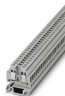
1,5 (1,5) mm 2 , 17,5 A, borne de paso
