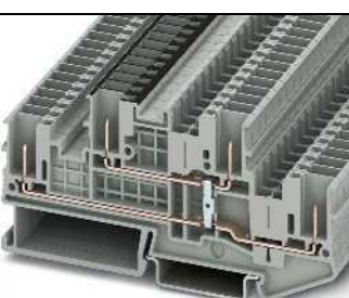
22 A, borne de doble piso con conexión de potencial
