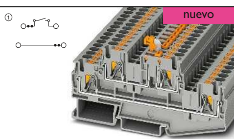
32 A, borne interrumpible por cuchilla de doble piso, una zona de interrupción
