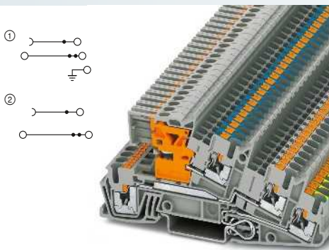
30 A, borne de tres pisos, 1 conductor exterior L, 1 conductor N seccionable, 1 x PE
