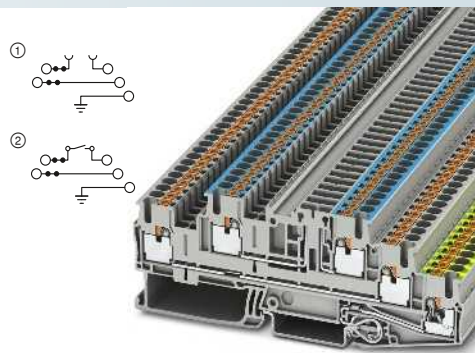
30 A, borne de tres pisos, con zona de interrupción y pie PE
