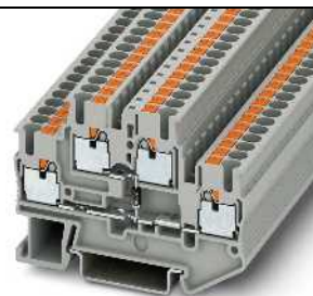
0,5 A, borne de doble piso de diodo, 1N 4007 (1300 V/0,5 A)
