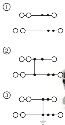
24 A, borne de doble piso, 3 conexiones por piso
