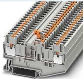
16 A, borne interrumpible por cuchilla, 4 fosos funcionales
