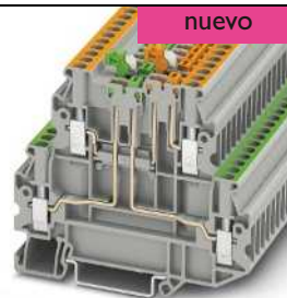
16 A, borne de doble piso con cuchilla seccionadora por piso
