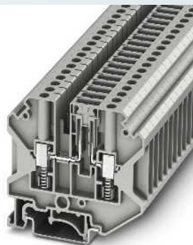
4 (6) mm 2 , 20 A, borne de separación, 2 conexiones
