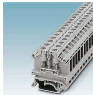
Bornes de conexión por espárrago para montaje sobre carril y montaje directo OTTA ...
