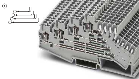
10 A, borne de cuatro pisos, dos slots
