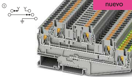
20 A, borne de tres pisos con zona de interrupción
