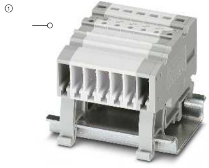
17,5 A, acoplamiento para montaje sobre carril
