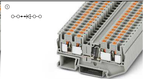
1,5 A, borne de diodo, 1N 5408 (1000 V/1,5 A)
