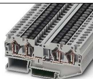
37 A, borne de paso, 4 conexiones, con yugo de corriente interrumpido
