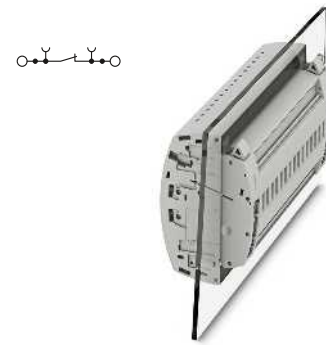
Regleta de clavijas de prueba 6 (10) mm 2 , 30 A, 4 ... 25 polos, para montaje mural, conexión push-in
