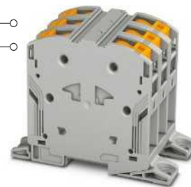
232 A, bloque de bornes para montaje directo
