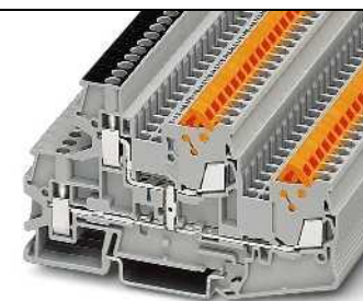
17,5 A, borne de doble piso con empalmador de potencial
