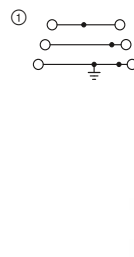
15 A, borne de varios pisos con pie PE
