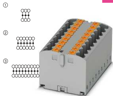
24 A, bloques de base, autoconfeccionables
