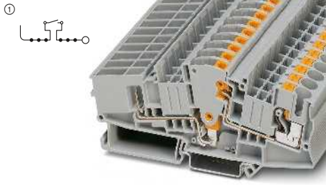
30 A, borne seccionable para transformadores de corriente, para conector de cortocircuito
