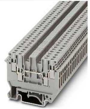
2,5 (4) mm 2 , 32 A, borne de paso, 4 conexiones
