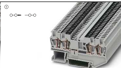
17,5 A, borne de paso, 4 conexiones, con yugo de corriente interrumpido
