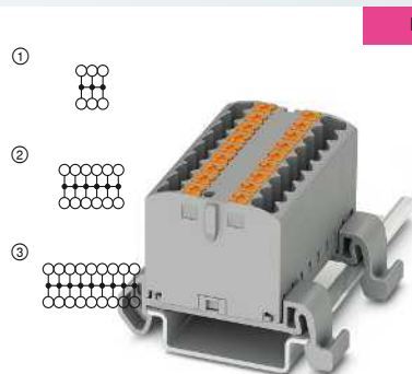
24 A, montaje sobre carril NS 35/7,5, longitudinalmente respecto al carril
