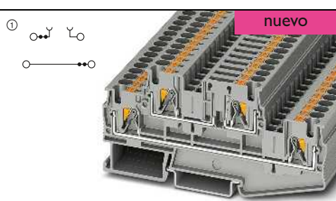
32 A, borne de doble piso, una zona de interrupción
