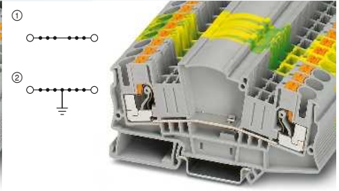
41 A, borne de paso, de igual contorno
