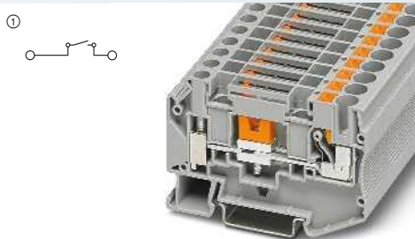
41 A, borne seccionable para transductores de medida
