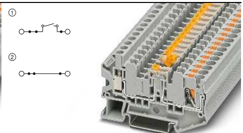
20 A, borne interrumpible por cuchilla, 3 fosos funcionales y dos conectores hembra de pruebas de 4 mm
