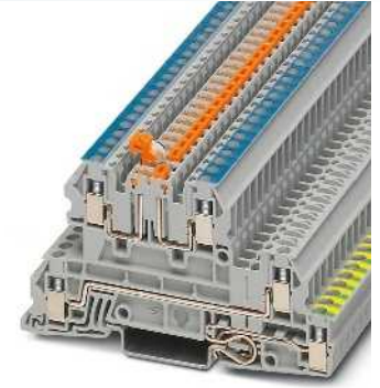
4 (4) mm 2 , 24 A, borne de tres pisos, 1 cable exterior L, 1 conductor N seccionable, 1 PE
