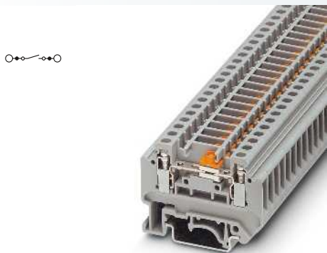
4 (4) mm 2 , 26 A, borne interrumpible para transductor de medida
