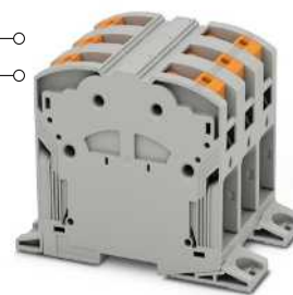
309 A, bloque de bornes para montaje directo
