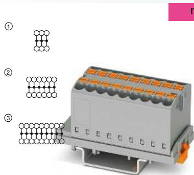
24 A, montaje sobre carril NS 35/7,5, transversalmente respecto al carril
