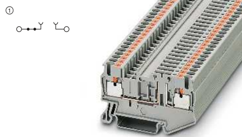
20 A, borne seccionable, con 2 fosos funcionales
