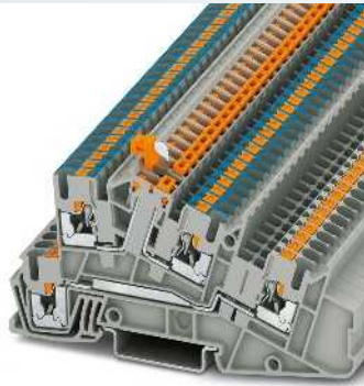
30 A, borne de tres pisos, 1 conductor exterior L, 1 conductor N seccionable
