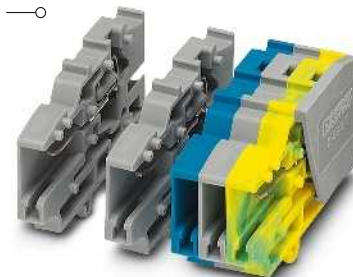
24 A, acoplamiento con espigas de encaje, autoconfeccionable
