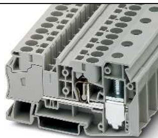
125 A (conexión por tornillo), borne colectivo de potencial, 4 entradas de 10 mm 2
