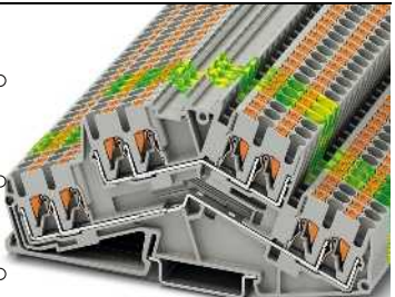
24 A, borne de doble piso, 4 conexiones por piso
