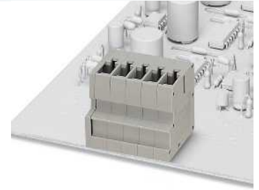
32 A, carcasa de base, sentido de conexión vertical
