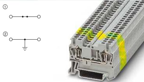
17,5 A, borne de paso
