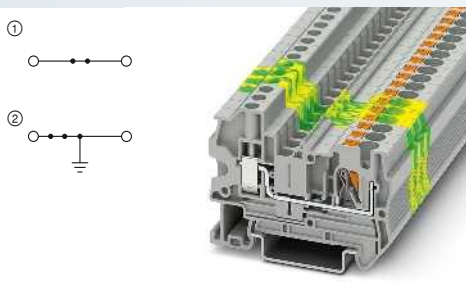
38 A, borne de paso
