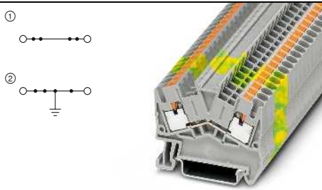
30 A, borne de paso
