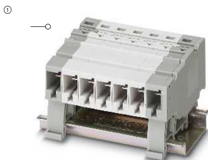
41 A, acoplamiento para montaje sobre carril
