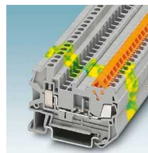
Bornes híbridos con conexión por tornillo en un lateral 1,5 mm 2 ... Pág. 206 2,5 mm 2 ... Pág. 210
