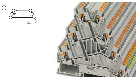
25 A, borne de cuatro pisos con pie PE
