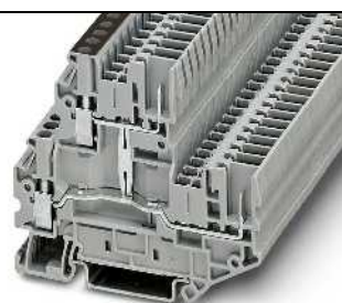
24 A, borne de doble piso con empalmador de potencial
