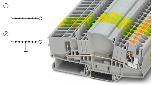
30 A, borne de paso, para conector de cortocircuito
