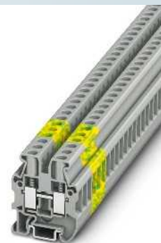
41 A, borne de paso y de tierra
