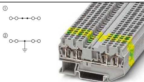
17,5 A, borne de paso, 4 conexiones
