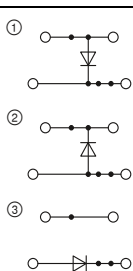
28 A, borne de doble piso de diodo, 1N 4007 (1300 V/0,5 A)
