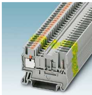
Bornes de paso, de varios conductores y de varios pisos así como bornes de tierra con conexión push-in 1,5 mm 2 ... Pág. 278 2,5 mm 2 ... Pág. 286 4 mm 2 ... Pág. 298 6 mm 2 ... Pág. 302
