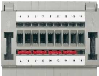
Regleta de clavijas de prueba para transformadores de corriente
