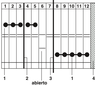
Borne interruptible por cuchilla URTK/SS
