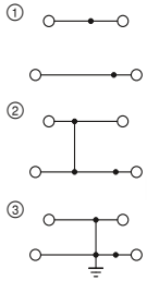
26 A, borne de doble piso, 4 conexiones
