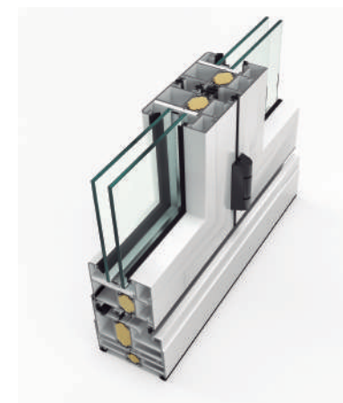
SERIE S72 RPT
