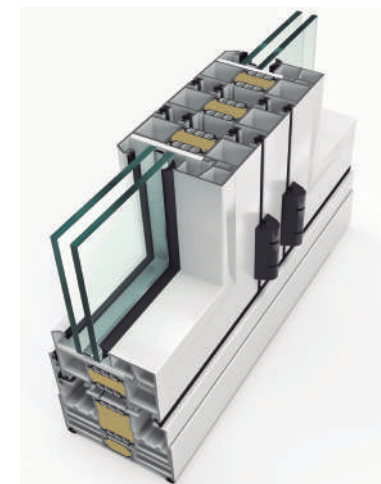
SERIE S112 RPT
