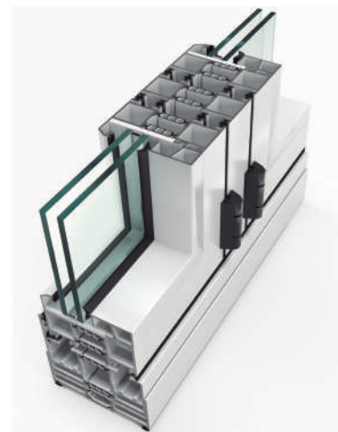
SERIE S110 RPT
