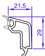
GAR7223 (FIJOS 24 MM)
