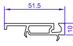
GAR7216 (ACOPLE JUNQUILLO FIJOS)
