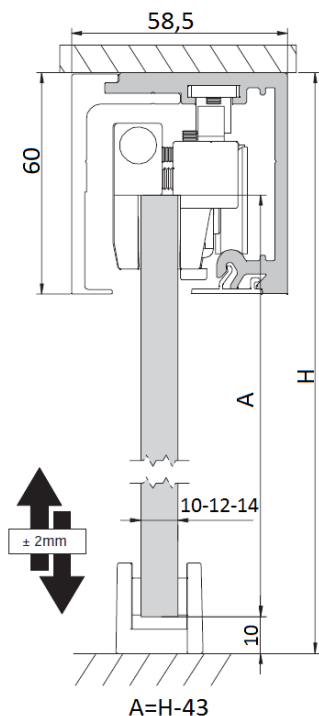
MONTAJE A TECHO
