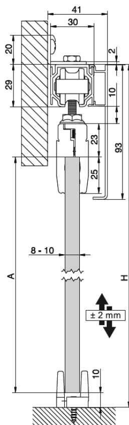
INSTALACIÓN A PARED
