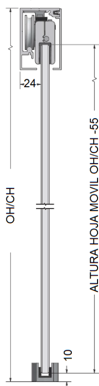
GUÍA E70 / ELEVA700
