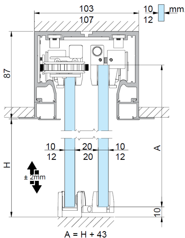
MONTAJE A VIDRIO FIJO
