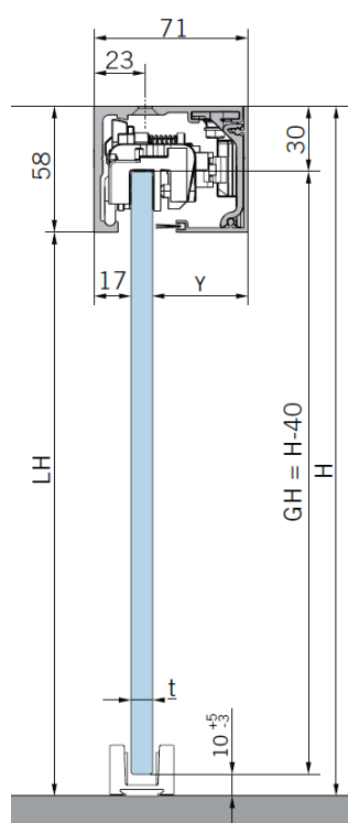
FIJACIÓN A TECHO
