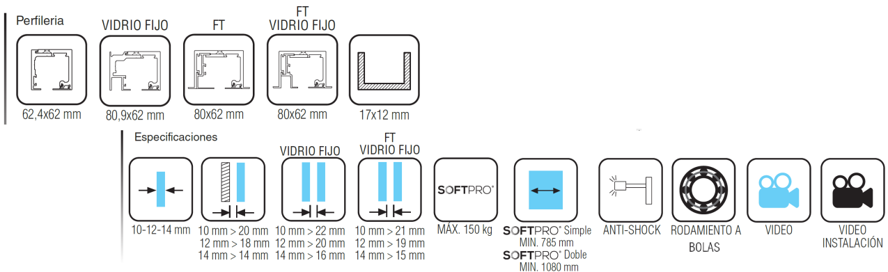
MONTAJE A PARED
