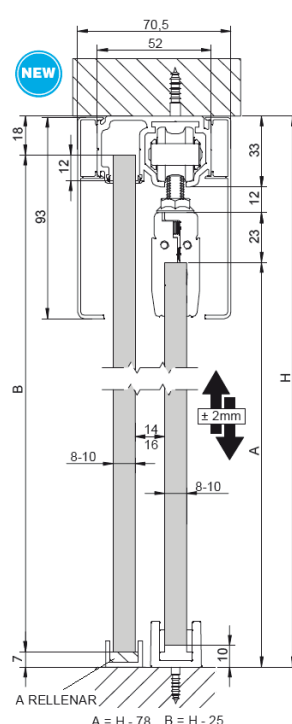
INSTALACIÓN A TECHO
