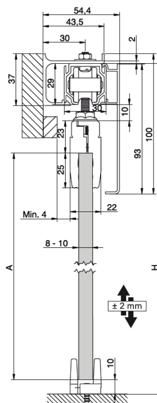
INSTALACIÓN A PARED CON PERFIL SEPARADOR
