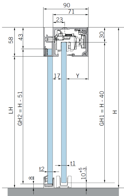
MONTAJE CON FIJO A TECHO
