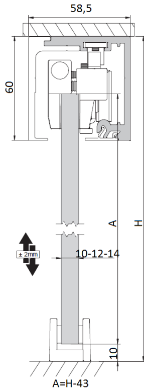
MONTAJE A TECHO
