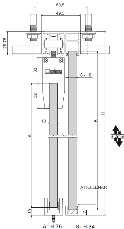
FALSO TECHO CON VIDRIO FIJO
