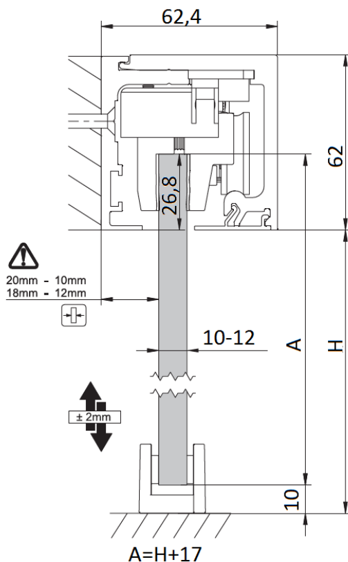
MONTAJE A PARED
