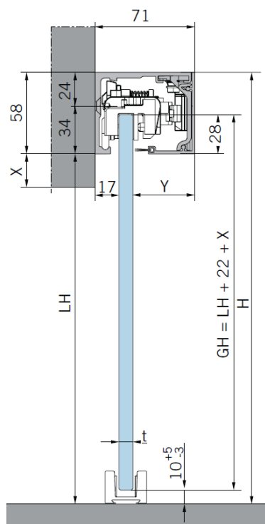
FIJACIÓN A PARED
