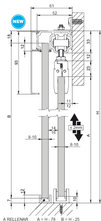
INSTALACIÓN A PARED
