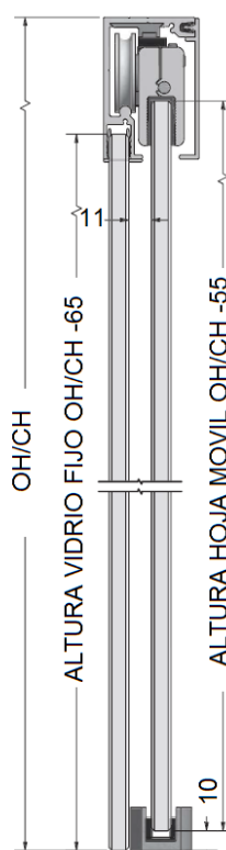
GUÍA CON FIJO
