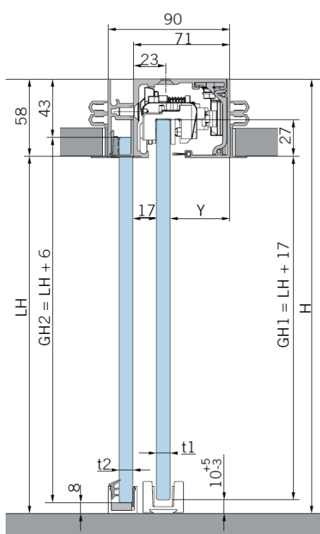
MONTAJE CON FIJO A FALSO TECHO
