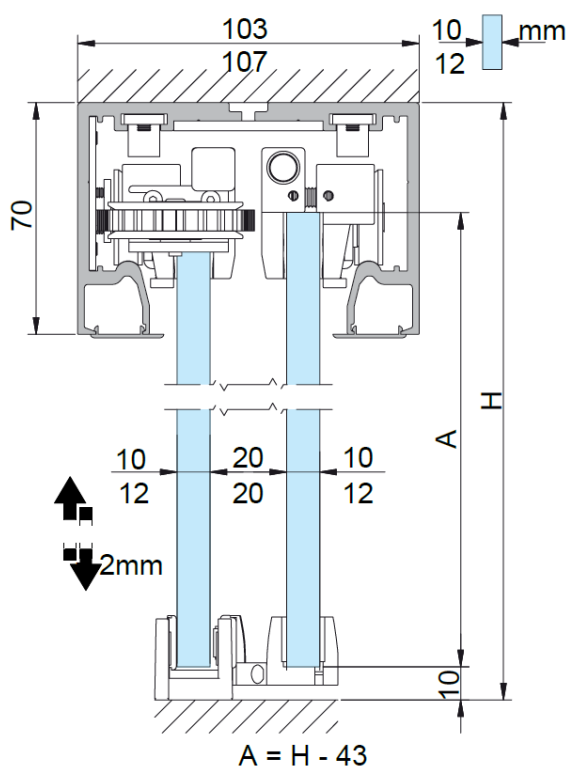
MONTAJE A TECHO
