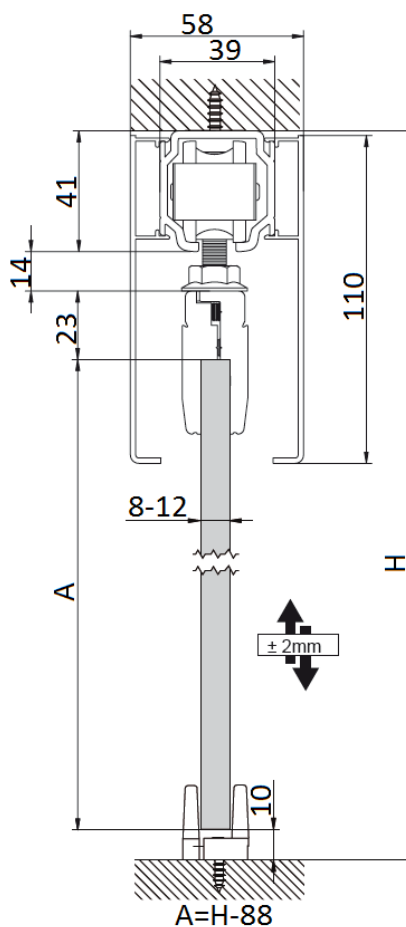
SV-A100 - INSTALACIÓN A TECHO
