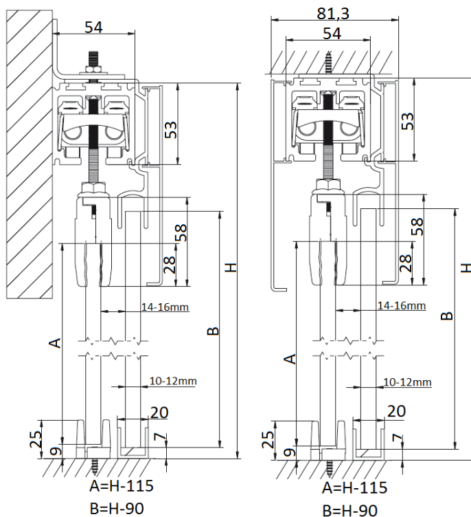
SV- A200 OPCIÓN VIDRIO FIJO
