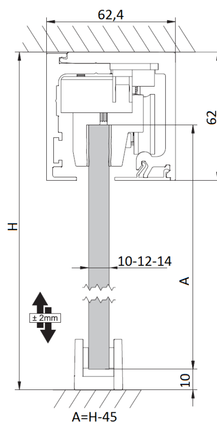
MONTAJE A TECHO
