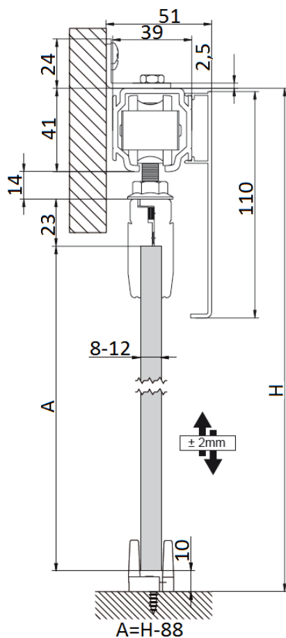
SV-A100 - INSTALACIÓN A PARED
