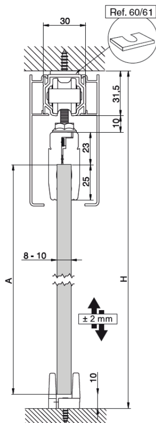
INSTALACIÓN A TECHO
