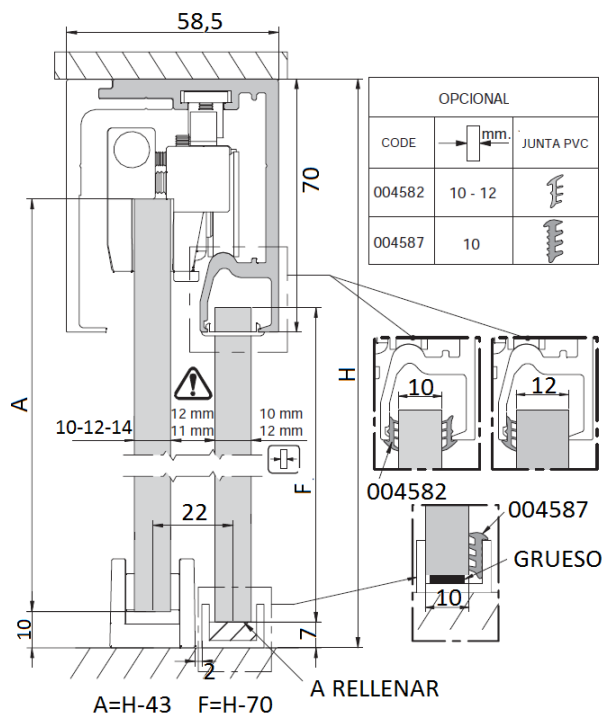
MONTAJE A TECHO VIDRIO FIJO
