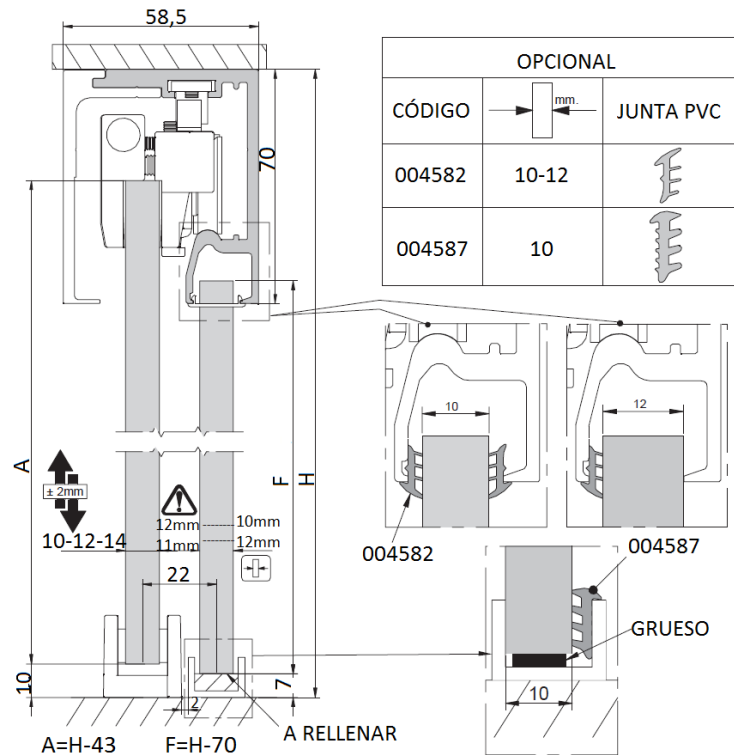
MONTAJE A TECHO VIDRIO FIJO
