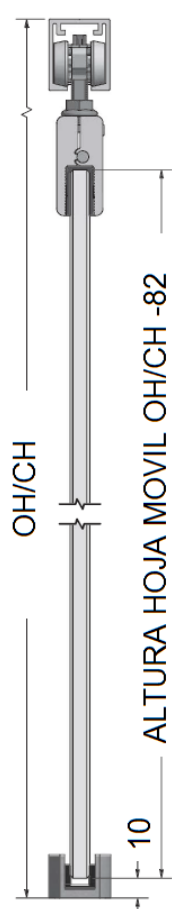
GUIA SIMPLE E200
