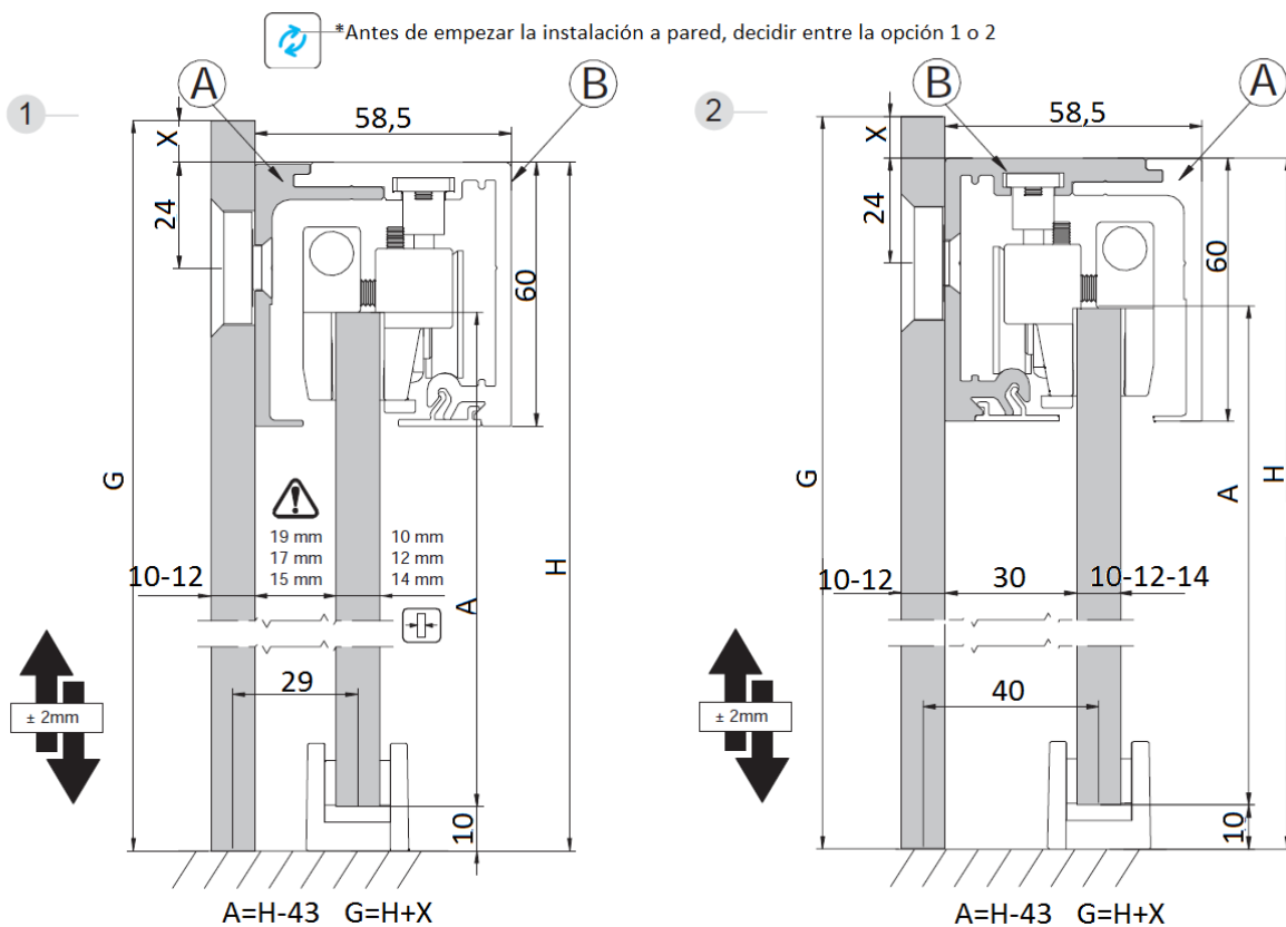
MONTAJE A PARED DE VIDRIO
