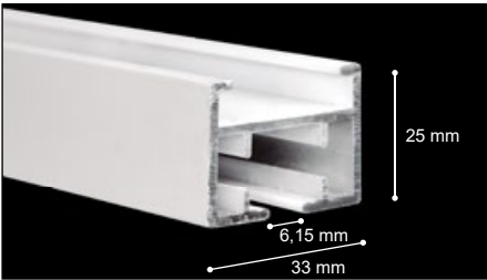
Perfil RM09
