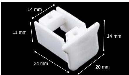
*Tapa *Encap / *Bouchon final
