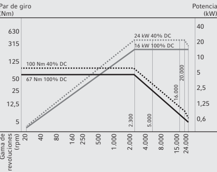
Motor husillo HSK-A63 24.000 rpm / 24 kW / 100 Nm
