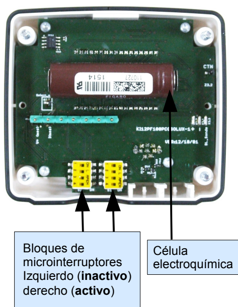
Interior de la parte frontal
