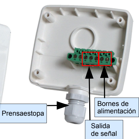
Parte trasera fija
