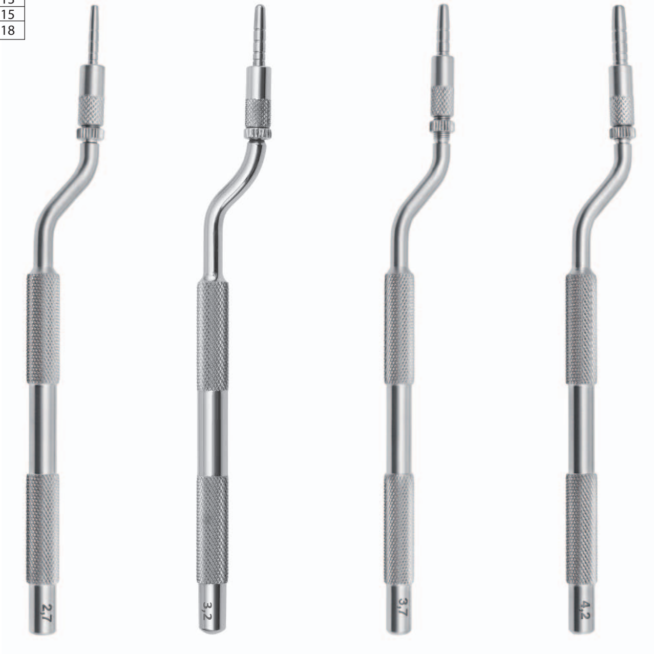
W119 Osteótomo. Elevador de senos con tornillo ajustable 2,7mm 59,00 €
