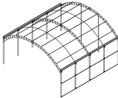
Estructura para 1 ó 2 Pistas
