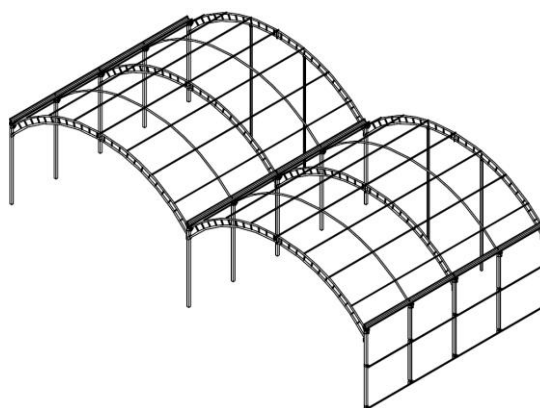
Estructura para 2 ó 4 pistas
