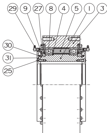
Design/Tipo 261 Form/Forma 1P
