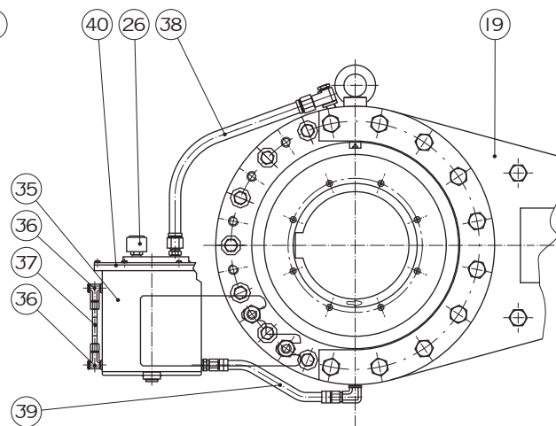
Design 261 with oil reservoir + torque arm Tipo 261 con depósito de aceite + brazo de torsión
