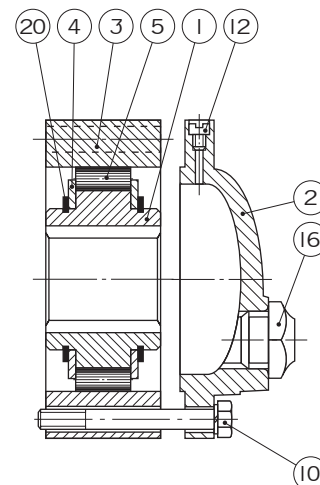
Design/Tipo 222
