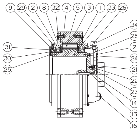
Design/Tipo 261 Form/Forma 2T
