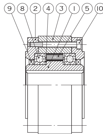
Design/Tipo 222
