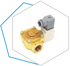
ELECTROVALVULA SMC 3/4" - 2V NC. LATON + BOBI- NA 24VAC 7W Y CONECTOR PRECIO EN WEB 51,40€
