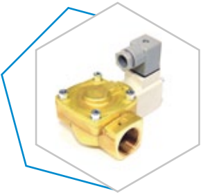
ELECTROVALVULA SMC 1" - 2V NC. LATON + BOBINA 24VAC 9W Y CONECTOR PRECIO EN WEB 64,32€
