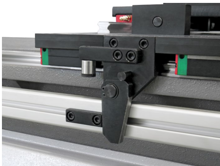
Topes magnéticos La distancia entre curvas (eje X) en las MDH-CN2 es definida a través de topes magnéticos.
