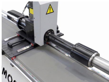
Mordaza del posicionador hidráulica El posicionador de control CN, está equipado con mordaza hidráulica.
