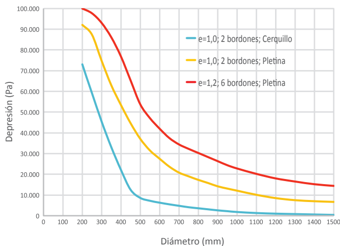
Depresión máxima permitida en función del diámetro del tubo
